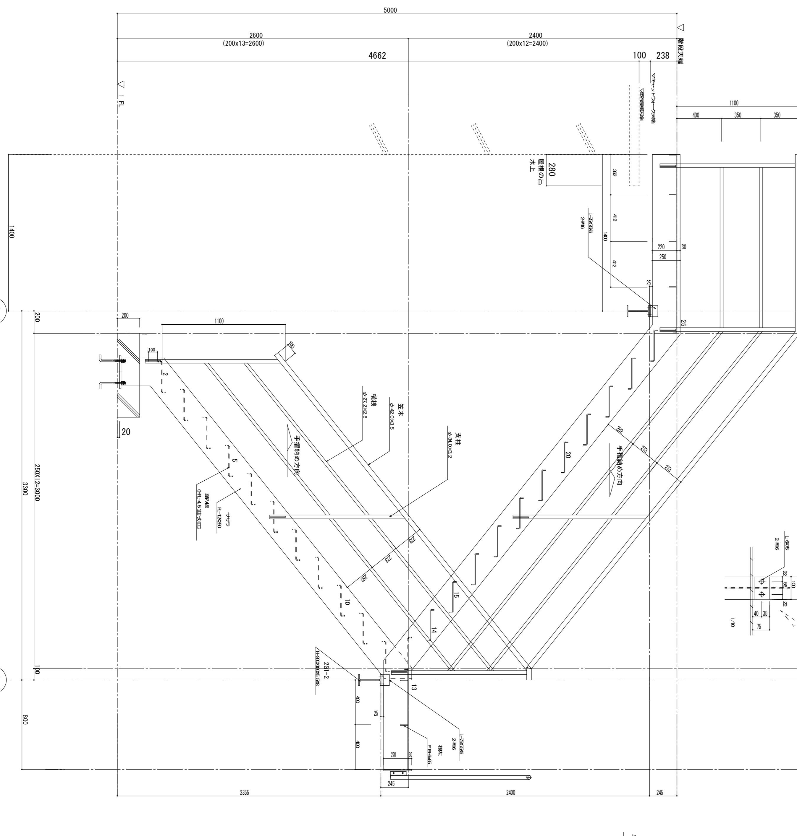
A-立面図
